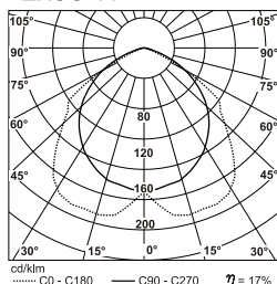
2x36 W
