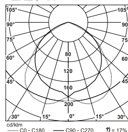
2x23 W
